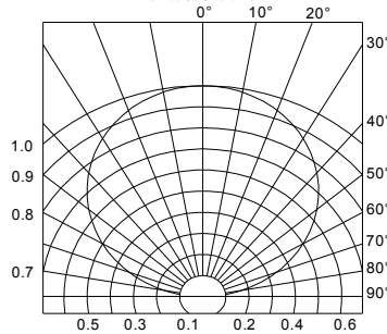
Radiation Diagram 辐射特性曲线
