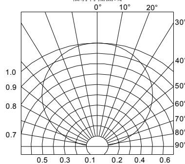
Radiation Diagram 辐射特性曲线
